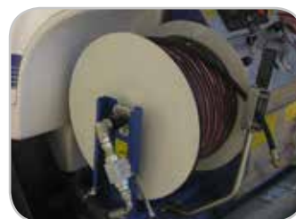
Naspo HP idraulico fisso + guida. Max tubo 100 mt 1/2" - 60 mt 3/4".
